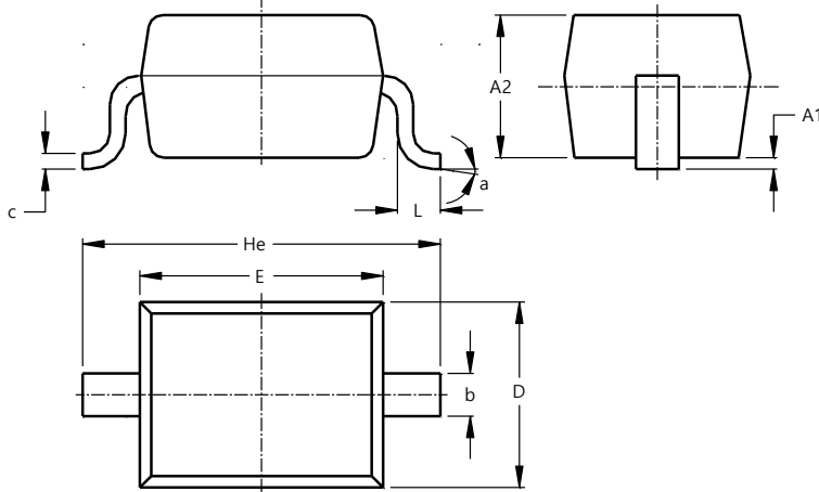
SOD323
