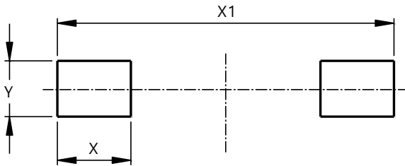
SOD323
