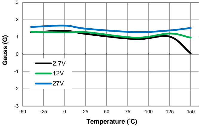
B MATCH (SP B OP - DIR B OP ) vs. Temperature
