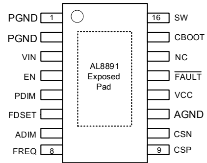
TSSOP-16EP
