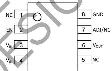
SOIC-8
