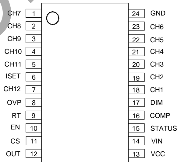
SOIC-24
