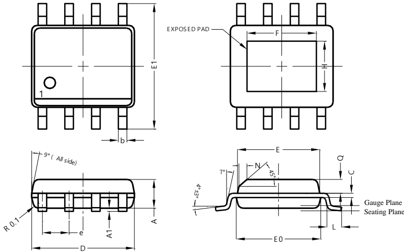
SO-8EP
