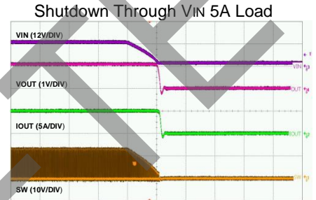
Time-200μs/div
