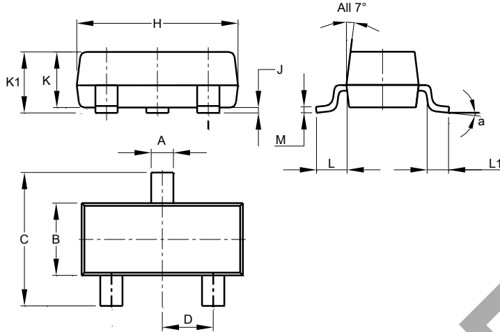
SOT23
