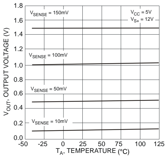
Fig. 6 Output Voltage
